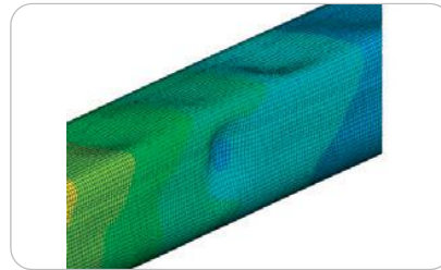
Bild 3: Beuluntersuchung am Teleskopausleger
