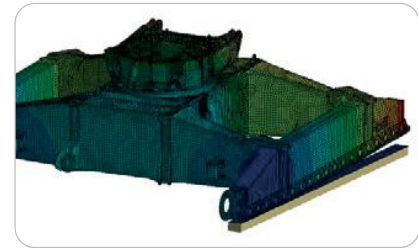
Bild 4: Raupenkranunterwagen
