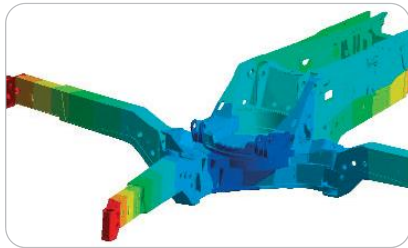
Bild 2: Verformungsuntersuchung an großer Unterwagen Baugruppe
